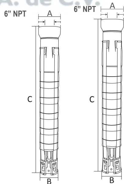
Acoplamiento NEMA 6" Fig. 1
